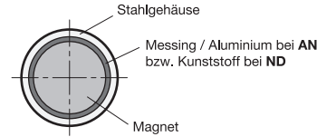
Ansicht auf Haftfläche
